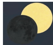
▲鹿嶋市から見える部分日食(予想)
