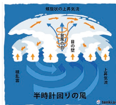
▲台風の構造の断面図 © 日本気象協会 tenki.jp
