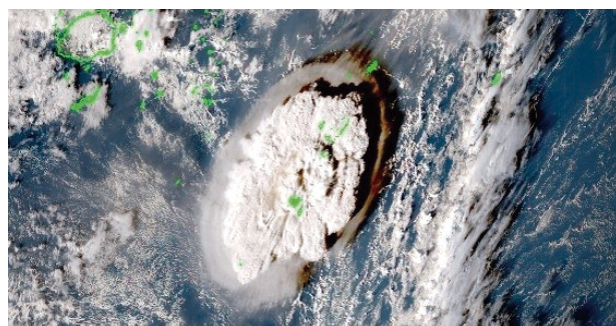
▲噴火直後の「ひまわり衛星」可視画像。
