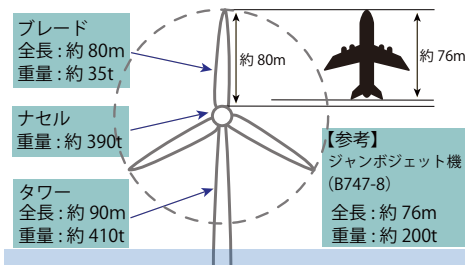
▲洋上風力発電設備の規模（8MW級） （出典：国土交通省資料）
