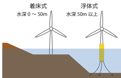
▲風車の構造形式 着床式と浮体式
