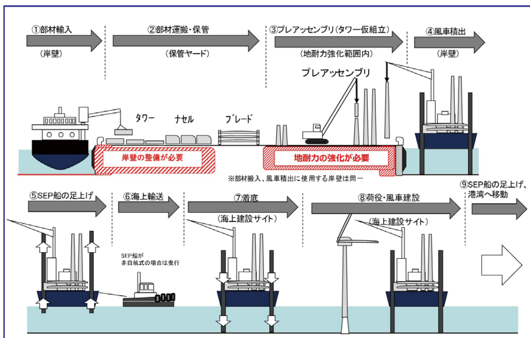
▲①部材輸入から②部材運搬や保管、③タワーの仮組立、④風車積出を行う「基地港湾」が鹿島港外港地区。SEP船(海上作業用の台船)に仮組立した風車などを乗せ、洋上風車を実際に設置する海域(=促進区域)まで輸送後、風車などの建設を行う。(出典：国土交通省資料)
